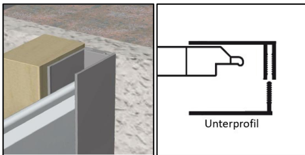
Zweiteiliges U-Profil
