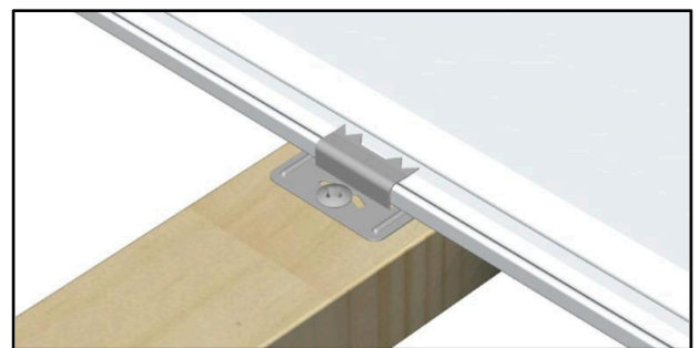
Befestigungsklammer
