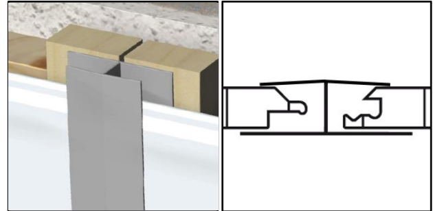
Einteiliges H-Profil
